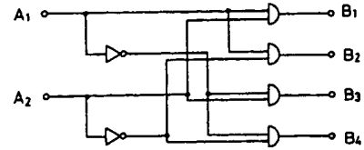
アドレスコード60の回路図 第5図
